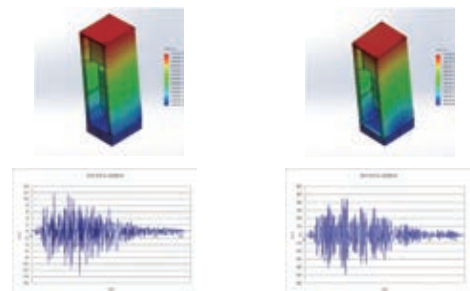
전후가진시 가진대에 대한 상단프레임 상대변위 좌우가진시 가진대에 대한 상단프레임 상대변위
