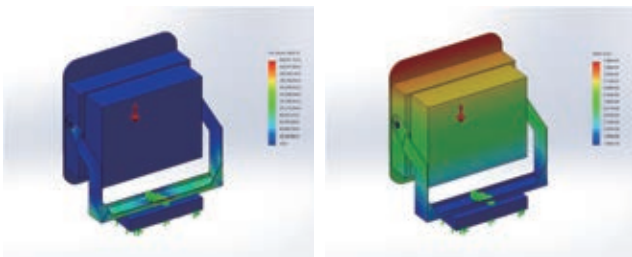
응력분포(Pa)
